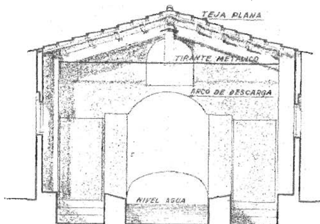
Plànol del "llavaner" D.G. "Regiones Devastadas"
